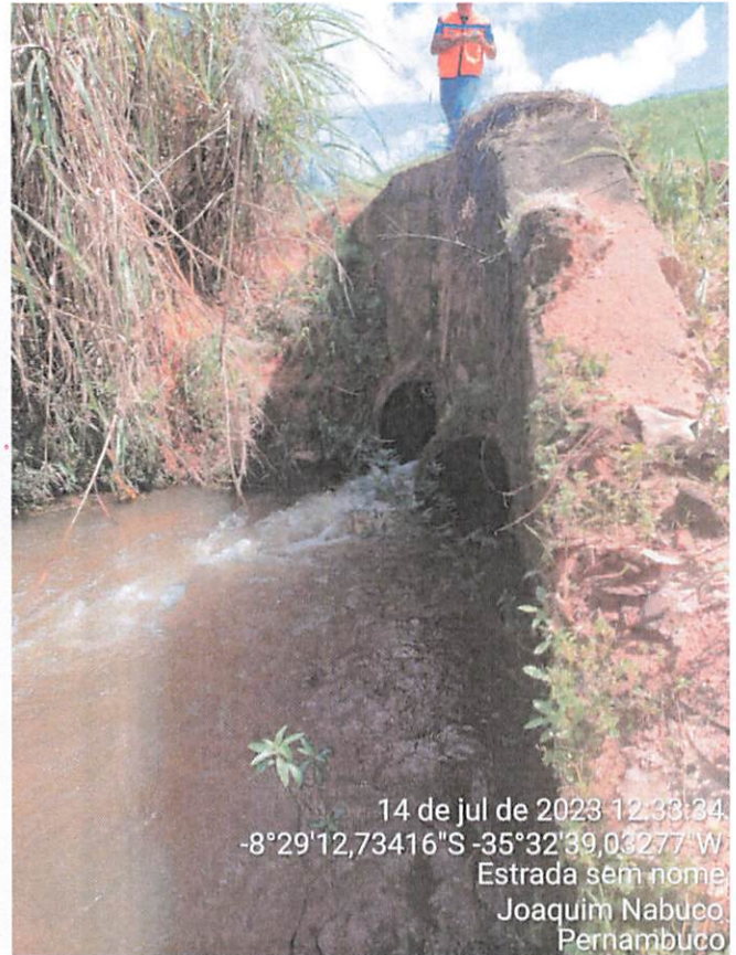
Imagem 02: Bueiro tubular de concreto com alas danificadas.
